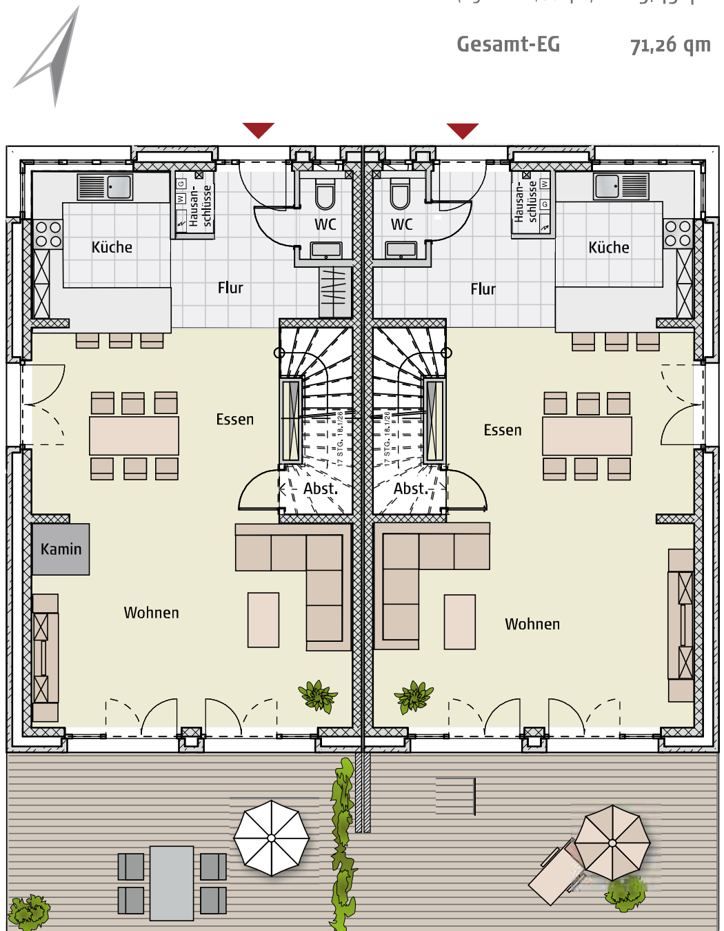
Grundrissvariante mit Sonderleistungen
